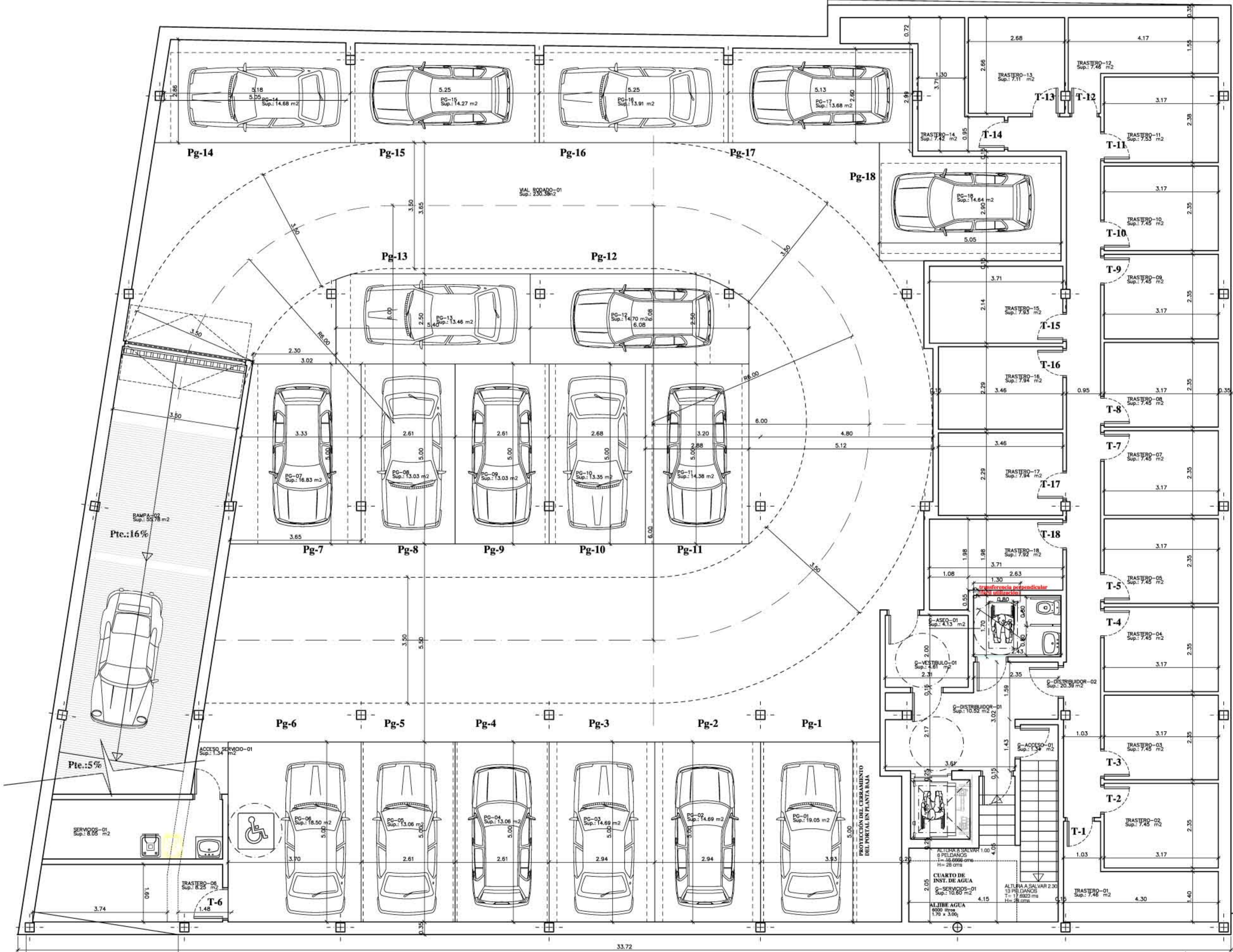
PLANTA DE GARAJE
